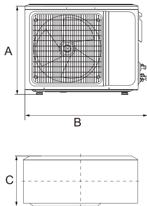
Fig.2 Unità esterna
